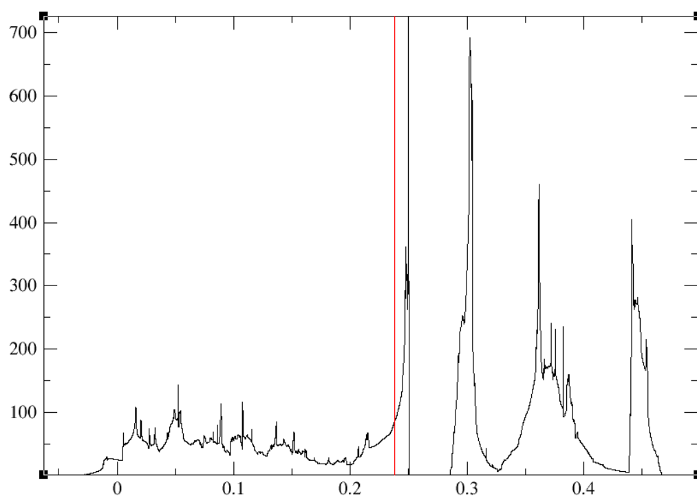
PBE0_O_pdos
