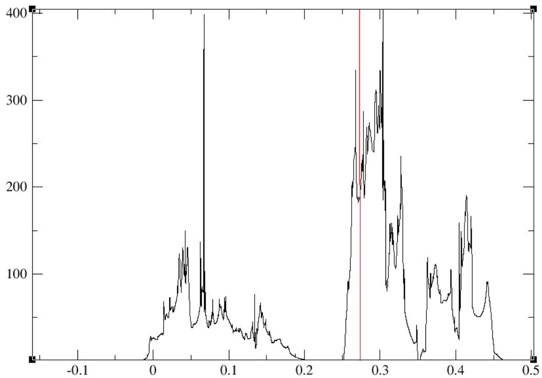
PAW_V_pdos
