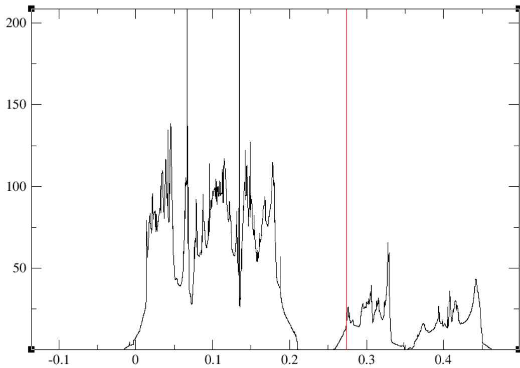
paw_O_pdos
