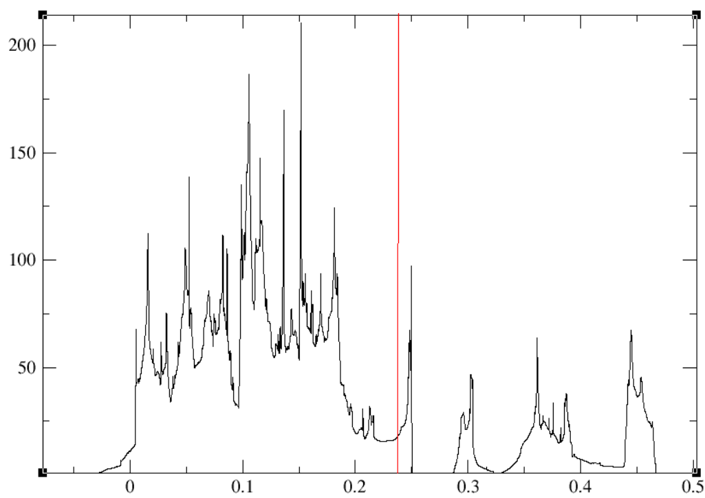
PBE0_O_pdos
